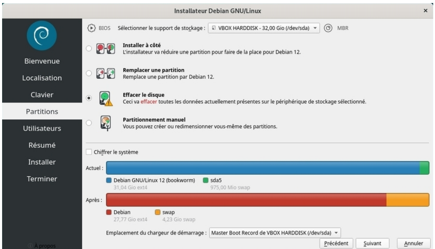
Installeur Calamares : schéma de partitionnement
