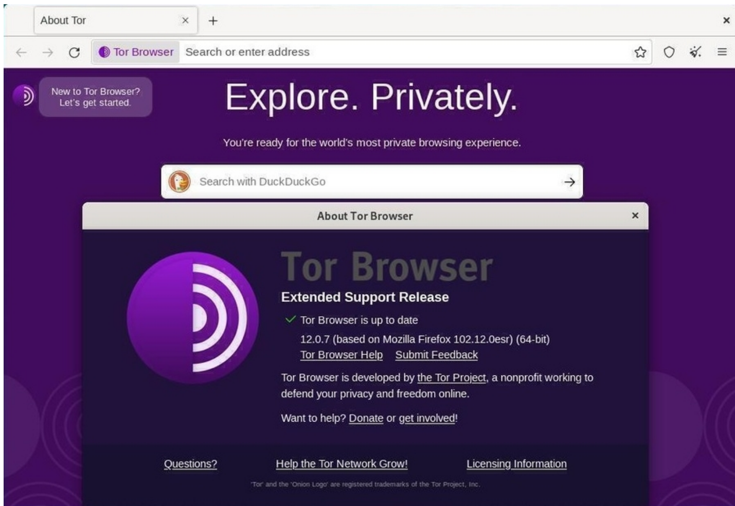
TorBrowser
