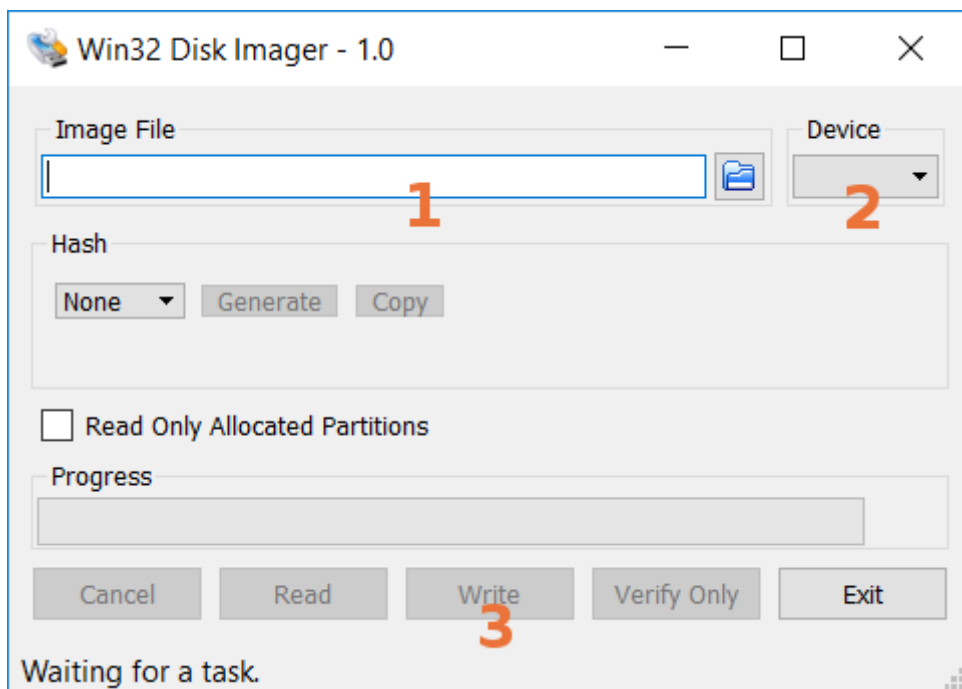
Win32DiskImager
